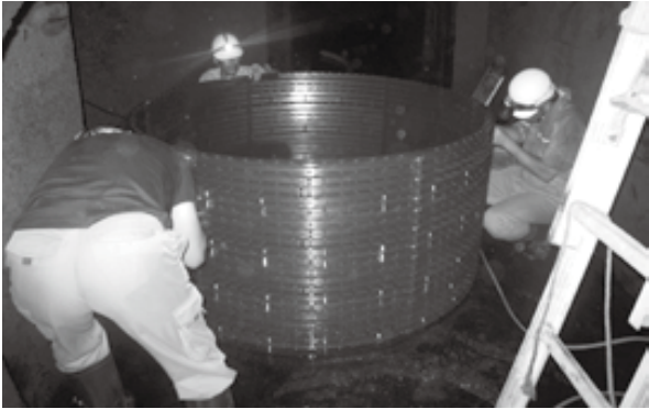
岳南3号第4排水路吐出管渠更生工事（製管工法） 管内での更生材組み立て状況
